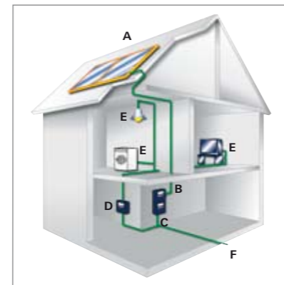
Alimentation photovoltaïque: A Élément de toiture photovoltaïque, B Onduleur, C Compteur de courant, D Compteur de consommation, E Consommateur, F Réseau public
