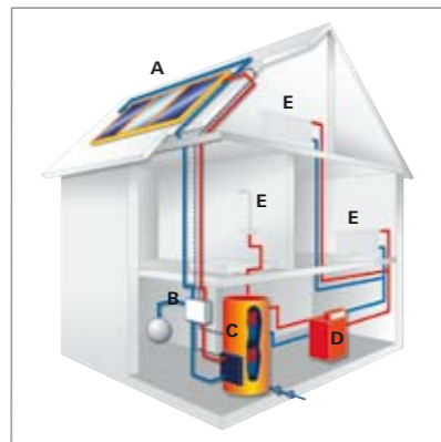
Alimentation thermique: A Élément capteur, B Poste de régulation solaire, C Accumulateur solaire, D Chaudière à gaz, à fioul (appoint), E Consommateur
